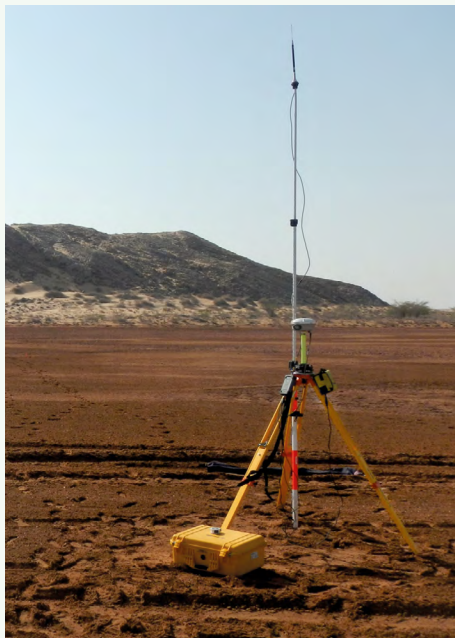
TotopographieOman : Relevés topographiques au GNSS Différentiel, Sultanat d'Oman / Crédit Adrien Barra
